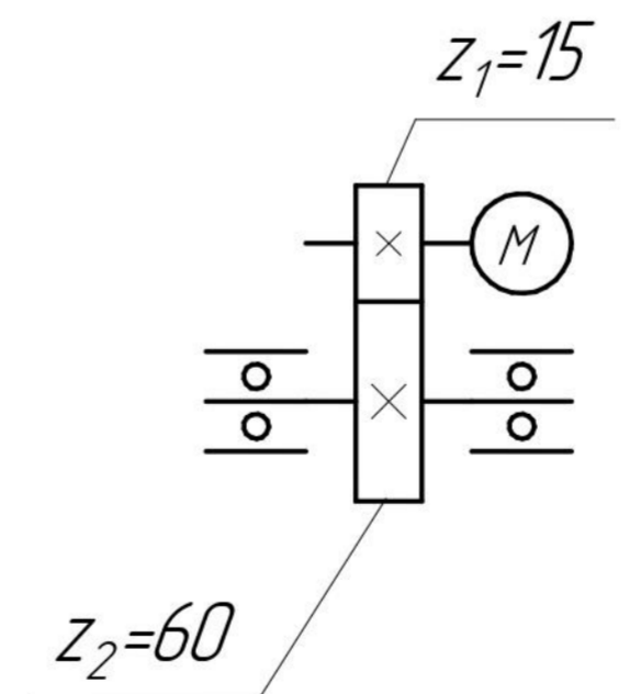
Кинематическая схема редуктора
